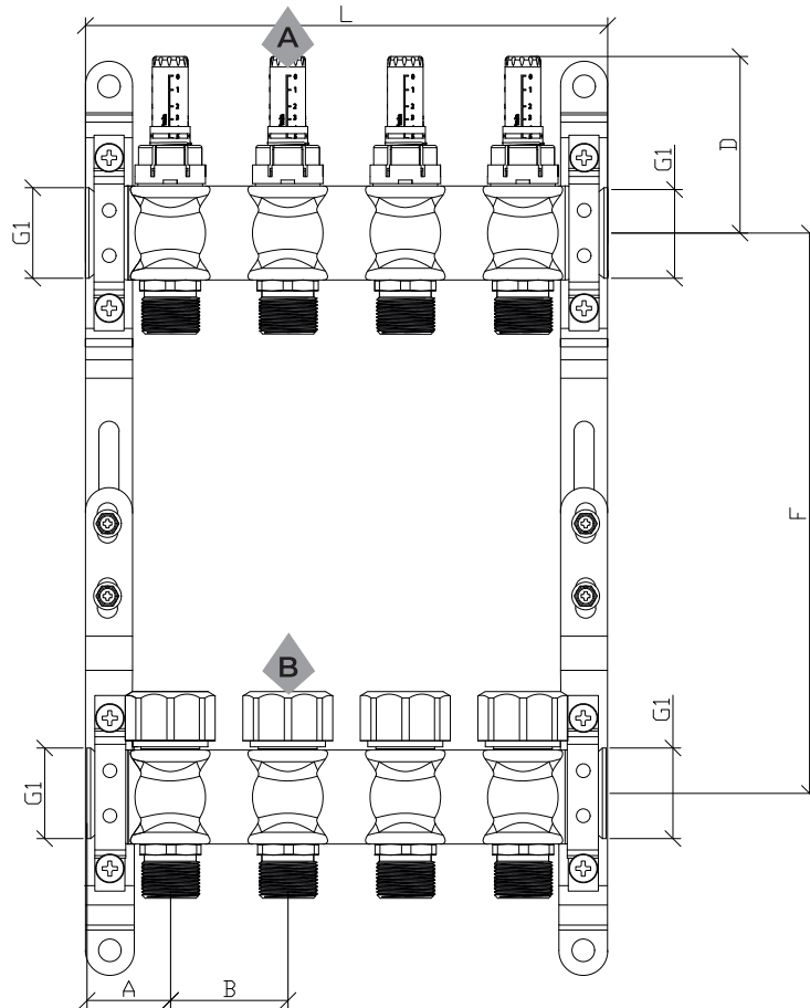
Kolektorový uzel s průtokoměry RCO3
