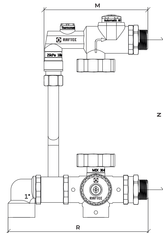
Gabaritní rozměry
